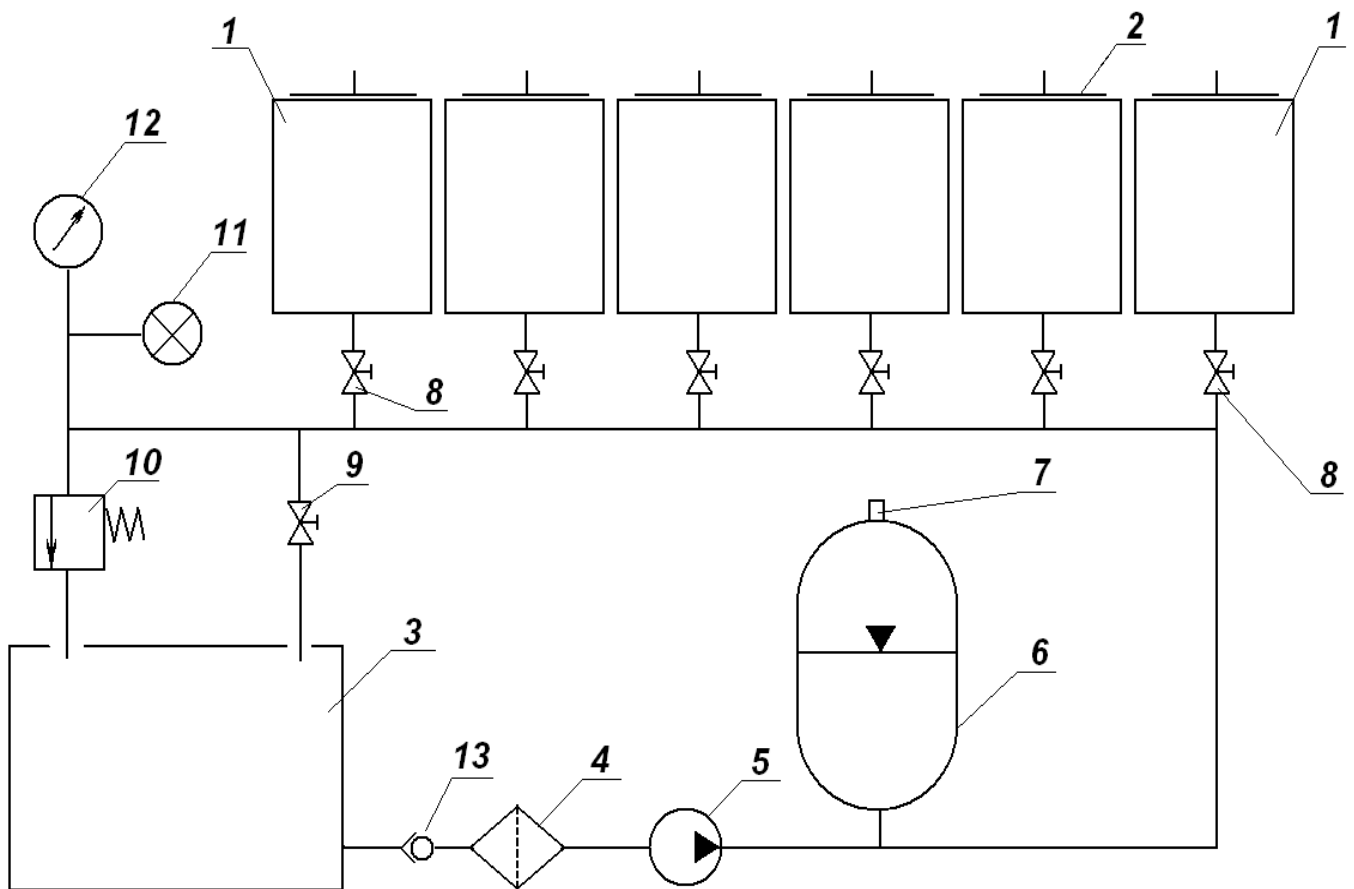
Рисунок 2 - Гидравлическая схема установки УВБ-МГ4.
