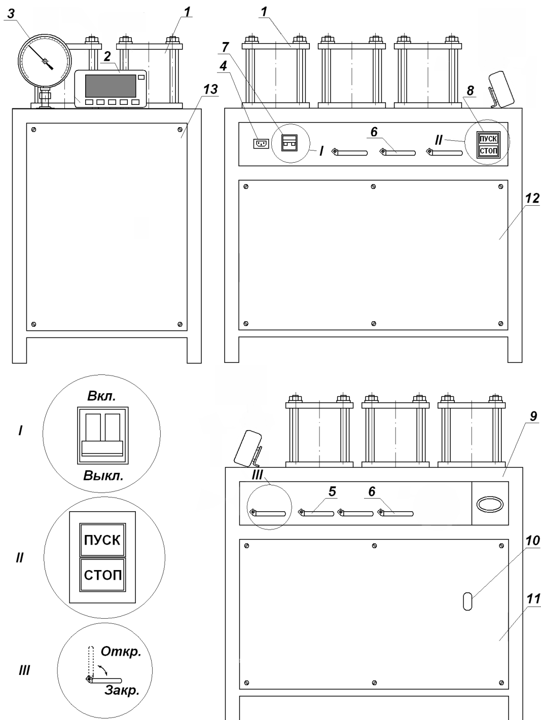
Рисунок 1 - Схема установки для испытания бетона на водонепроницаемость УВБ-МГ4 (УВБ-МГ4.01).
