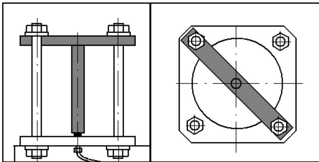
Рисунок 12 - Установка приспособления для проверки герметичности трубопроводов.
