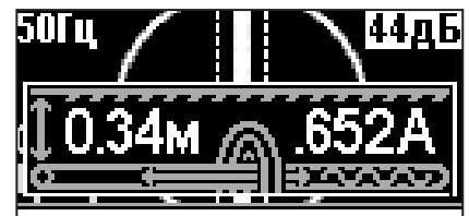
Ось трассы и ось прибора совпадают, доступно измерение глубины и тока в коммуникации.
