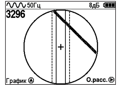
Положение указателя трассы показывает, в каком направлении от оператора находится коммуникация.
