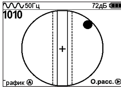
Наличие «шарика» показывает присутствие коммуникации на значительном удалении от оператора.
