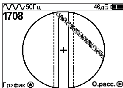
При искаженном поле сигнала отображается «размытая» линия указателя трассы.
