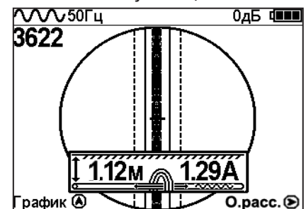
Ось коммуникации и ось прибора совпадают, доступно измерение глубины и тока в коммуникации.
